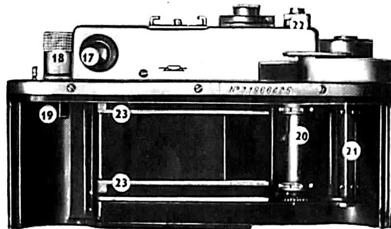
Рис. 3. Вид сзади со снятой крышкой. 17—окуляр видоискателя и дальномера; 18—головка обратной перемотки; 19—поводок кассетной катушки; 20—мерный валик; 21—приемная катушка; 22—втулка отключения затвора; 23—ползки фильмового канала
