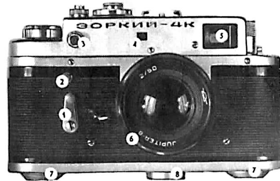
Рис. 1. Вид спереди. 1—рычаг автоспуска; 2—кнопка включения автоспуска; 3—штепсельный разъем для лампы-вспышки; 4—окно дальномера; 5—окно видоискателя и дальномера; 6—объектив; 7—замки съемной крышки; 8—штативная гайка
