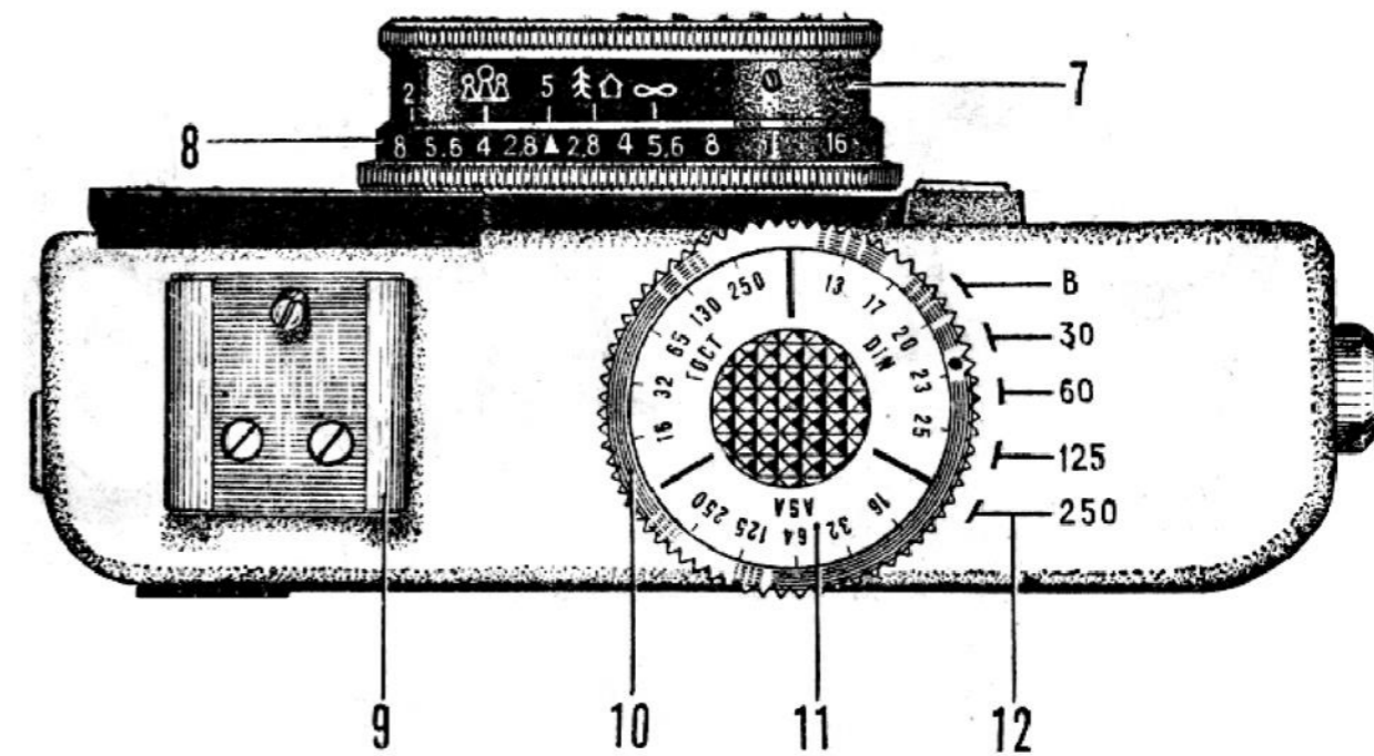
Рис. 2. Вид сверху.
