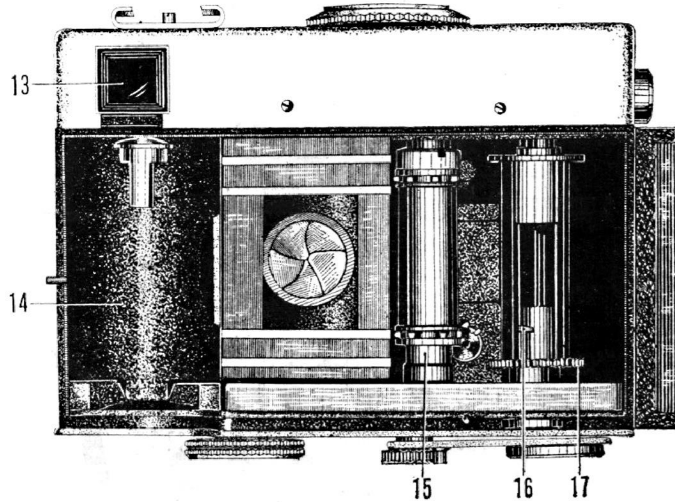
Рис. 3. Фотоаппарат с открытой задней крышкой
