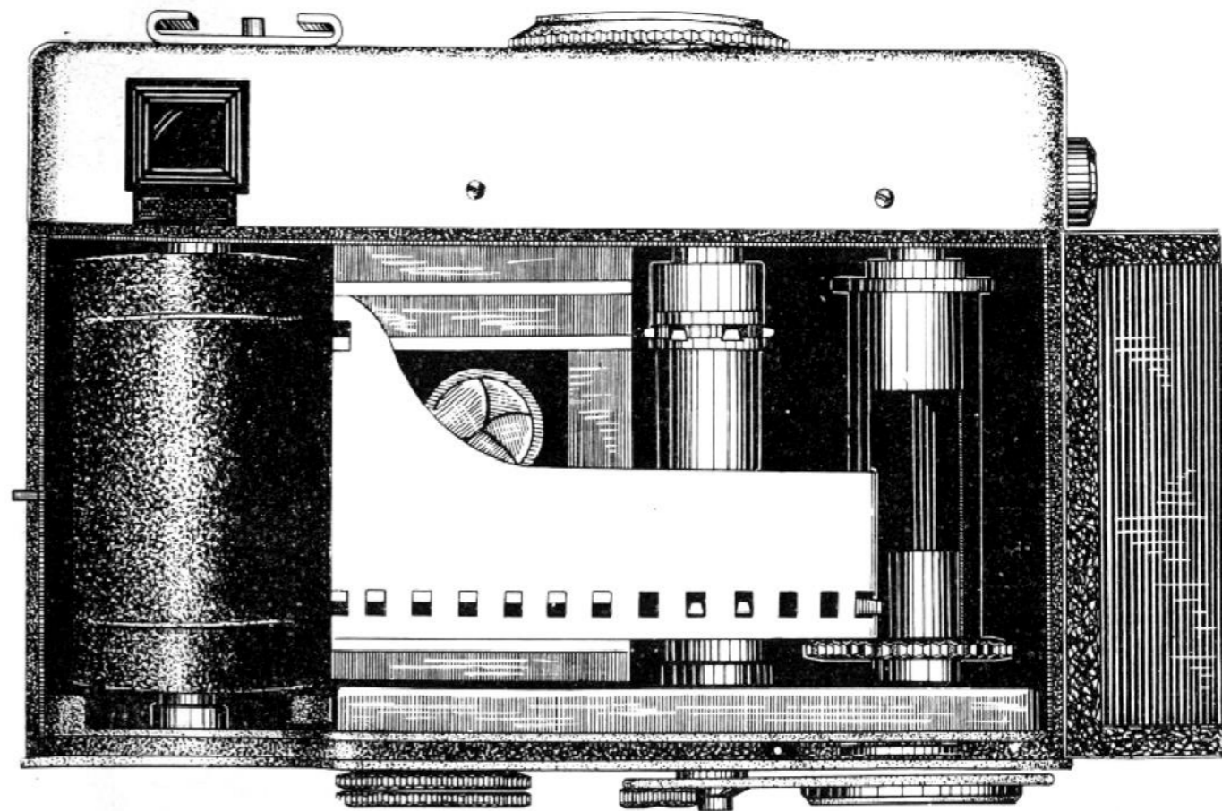
Рис. 8. Фотоаппарат с заряженной кассетой.
