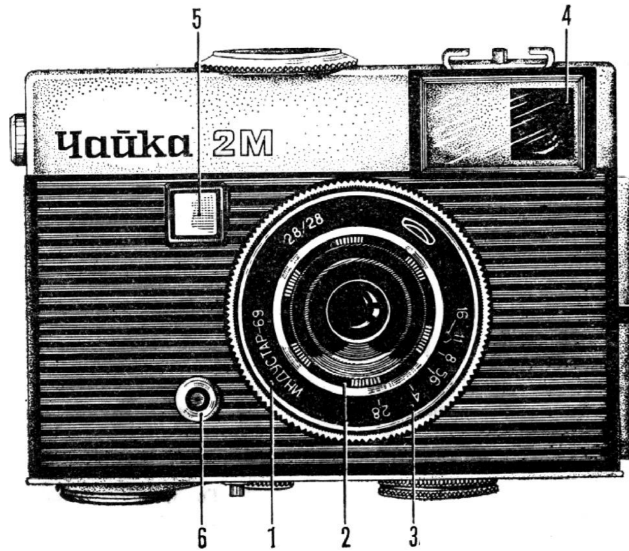
Рис. 1. Вид спереди.
